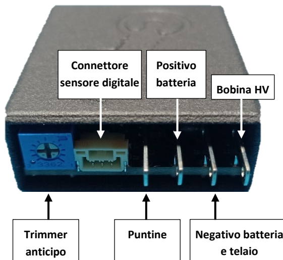
Figura 1: Vista frontale
